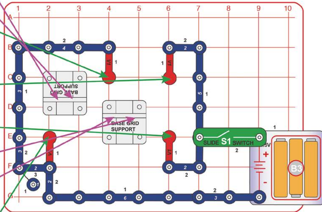
Pohľad zhora
