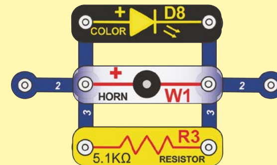
Paralelní obvod
